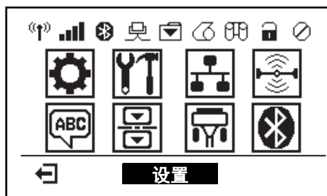
图 7 • 主菜单
