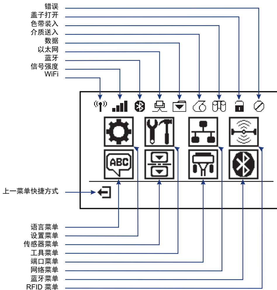
图 5 • 主菜单
